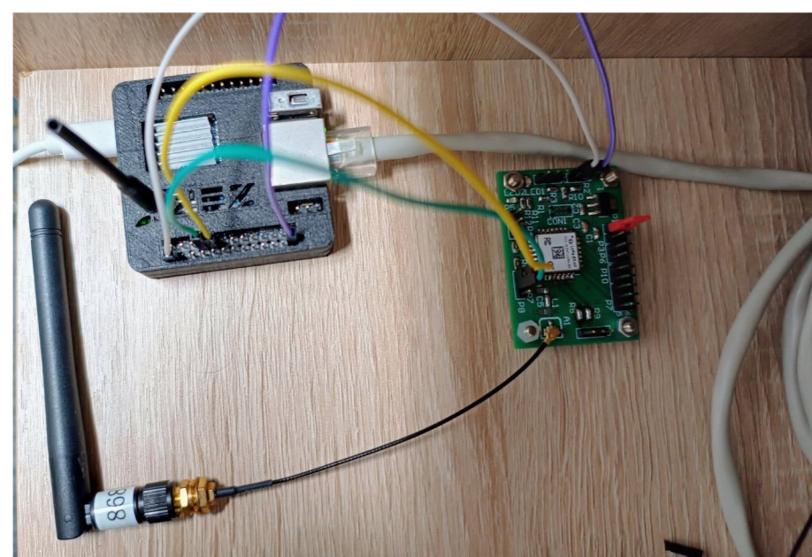
LoRa brána + Orange Pi
