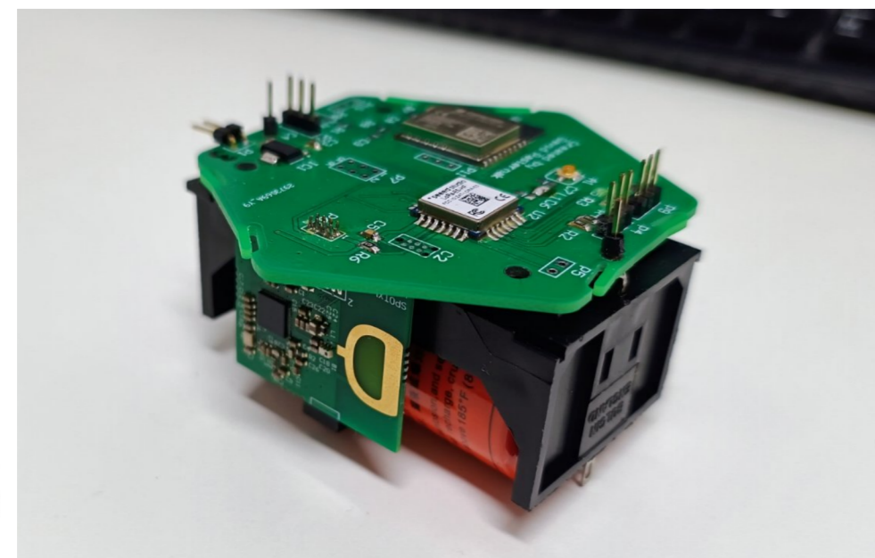
LoRa koncové, lokalizačné zariadenia s UWB technológiou
